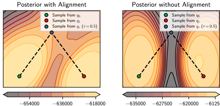
Figures 2/3: Posterior visualization.
