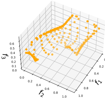
(d) Agg-Tche
