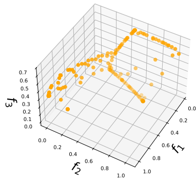
(g) Agg-SoftTche
