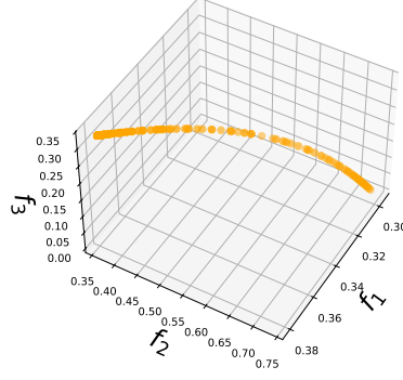
(e) EPO
