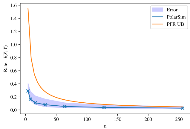
AWGN \sigma = 0.5
