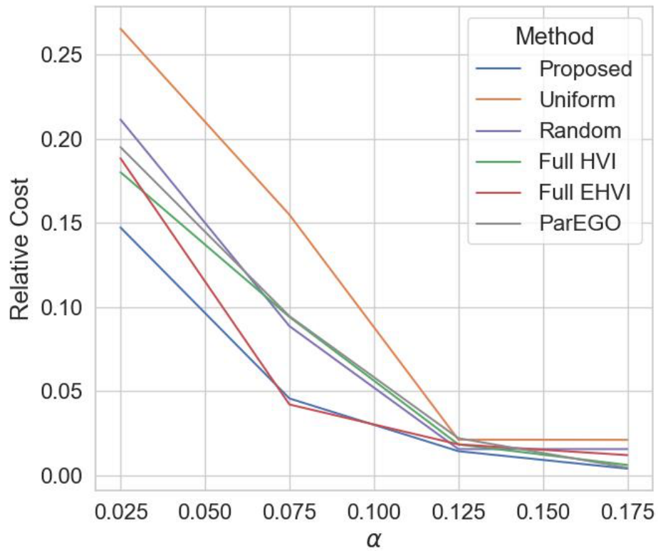
(d) Pruning
