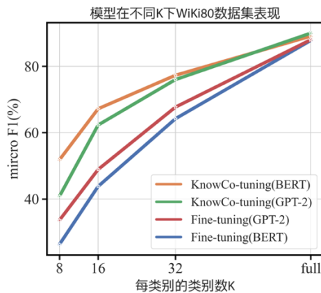
Fig.3 Experiments results based on GPT2 and BERT 图 3 基于 GPT2 和 BERT 的 KnowCo-Tuning 实验结果
