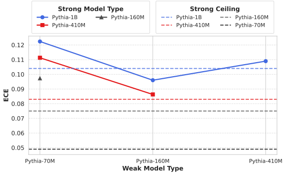
(c) ECE (Pythia).
