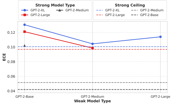
(d) ECE (GPT-2).
