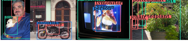
Meta Yolo
