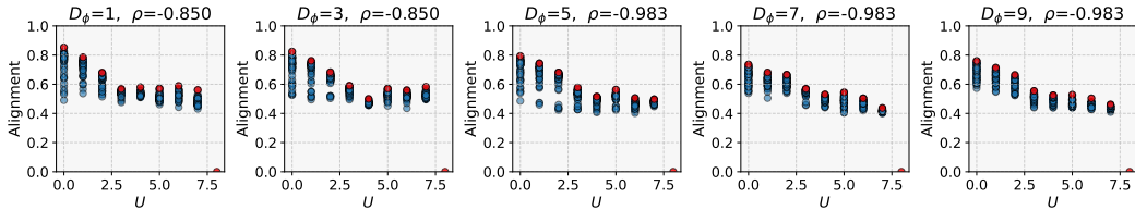
(d) Mutual k -NN ( k = 100 ), Batch Size = 256
