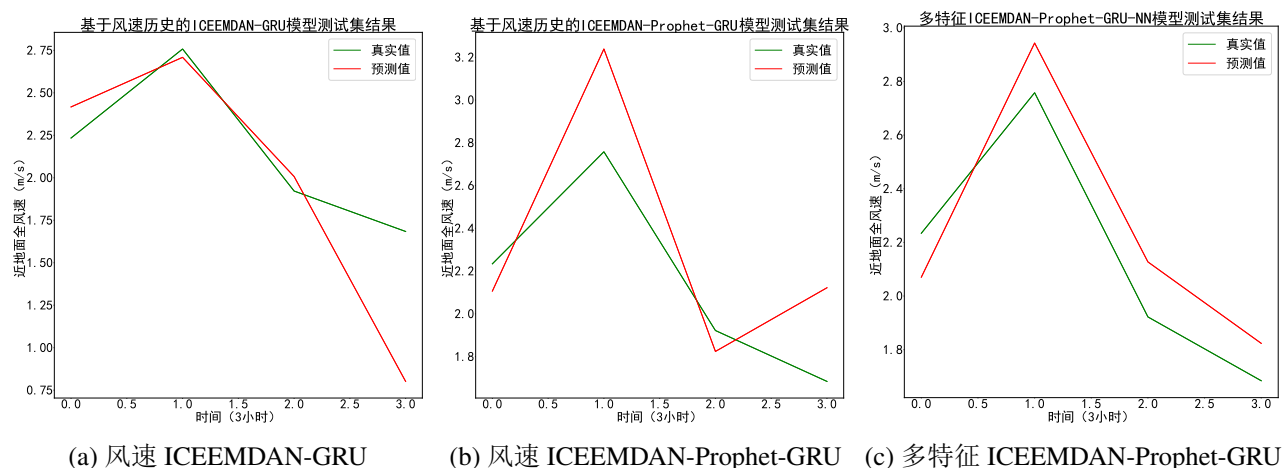
图 4.13 三种基于本文提出的神经网络的模型四步预测（12 小时）风速的可视化图
