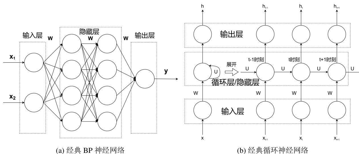
图 3.2 两种经典神经网络结构示意图
