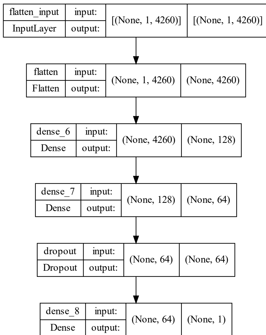
图 4.11 多特征 ICEEDMAN-Prophet-GRU-NN 模型中使用的 NN 模型网络结构图
