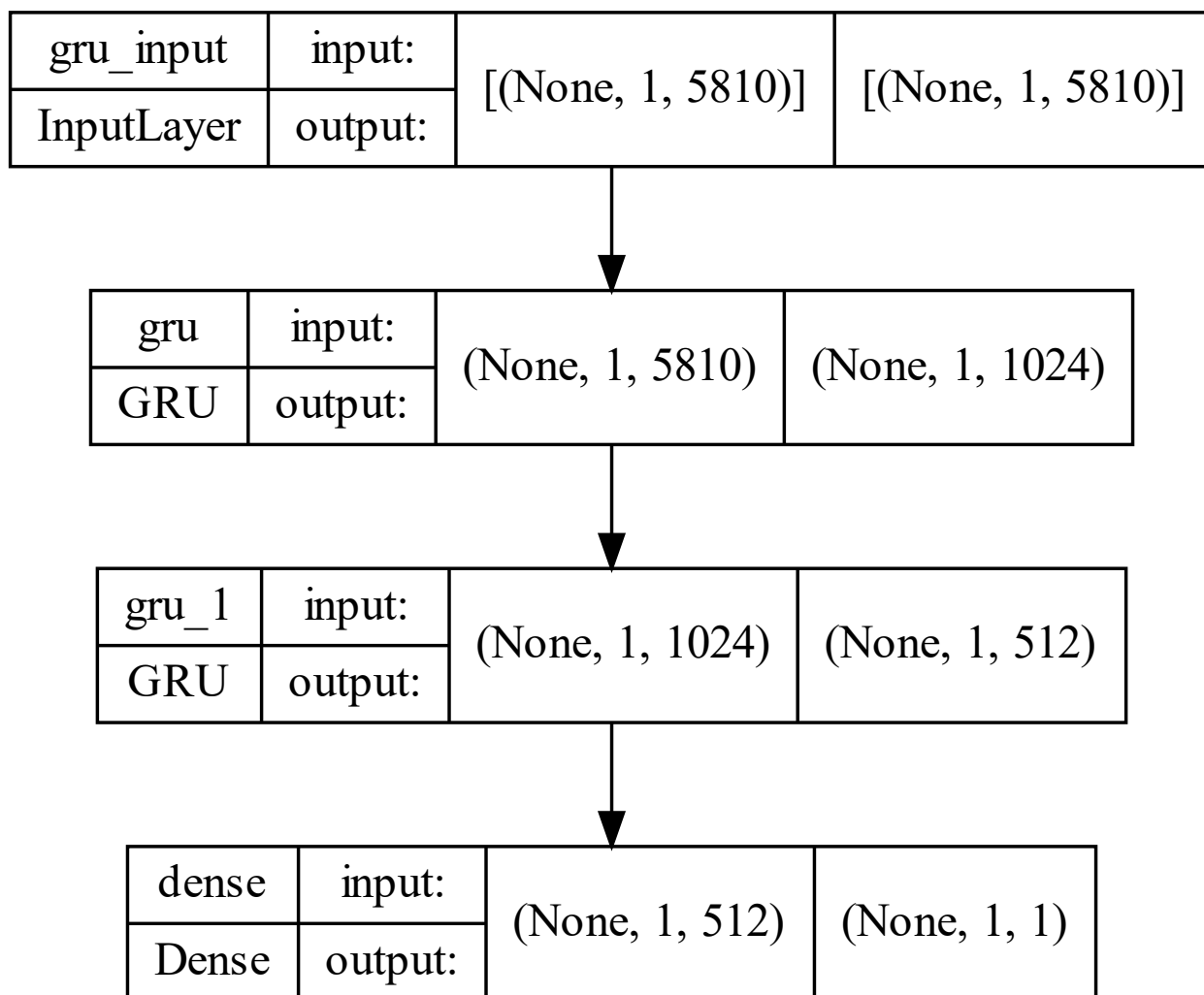
图 4.8 本文使用的 GRU 模型网络结构图
