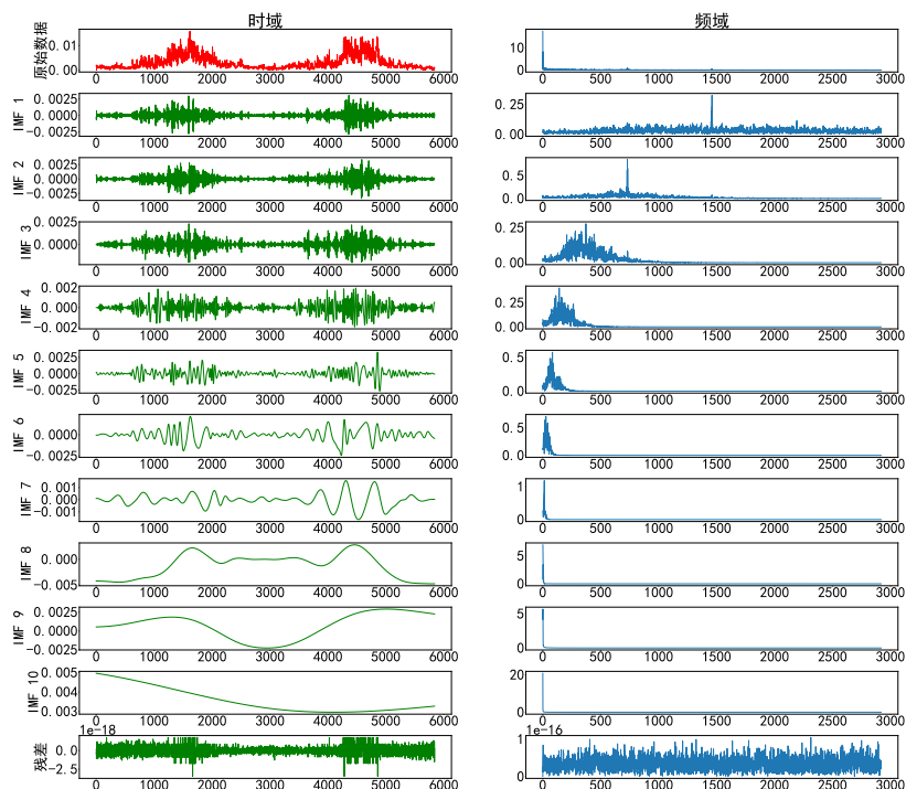
图 4.3 近地面空气相对湿度原始数据、ICEEMDAN 分解 IMF 分量、残差（左）及对应幅频图（右）
