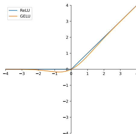
图 3.5 ReLU 和 GELU 函数图像
