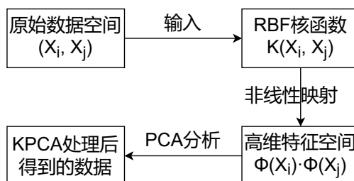
图 3.1 基于 RBF 的核主成分分析算法工作流程示意图
