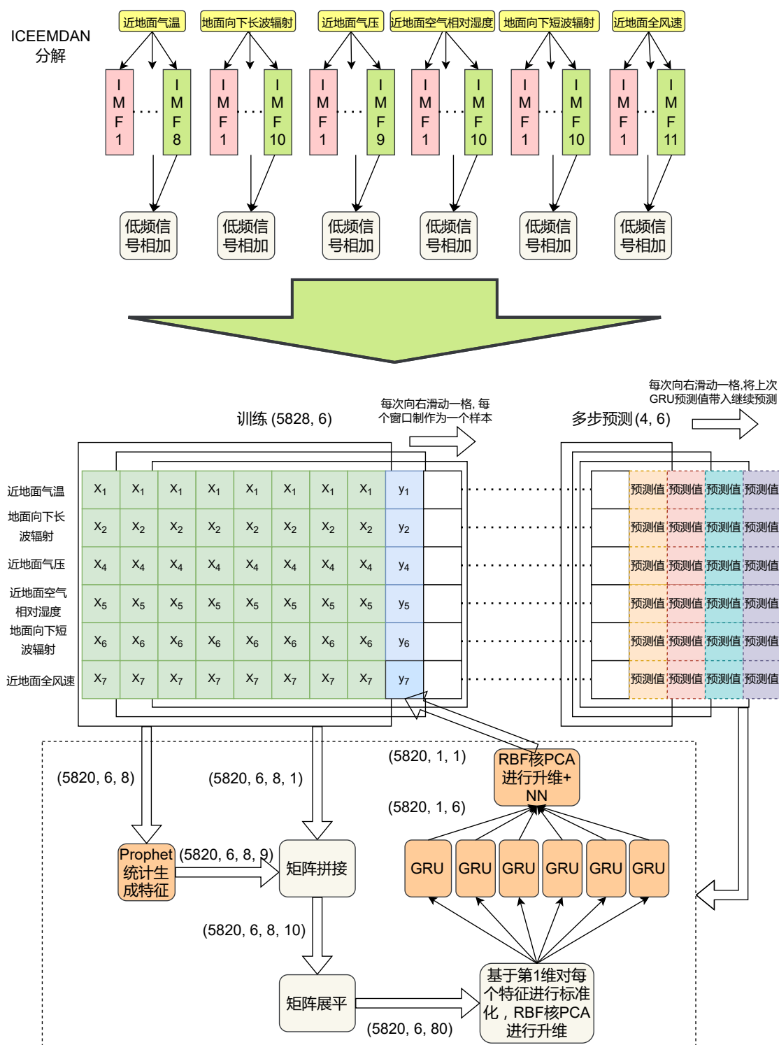
图 4.10 多特征 ICEEMDAN-Prophet-GRU-NN 模型结构图
