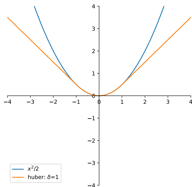
图 3.8 huber 函数图像
