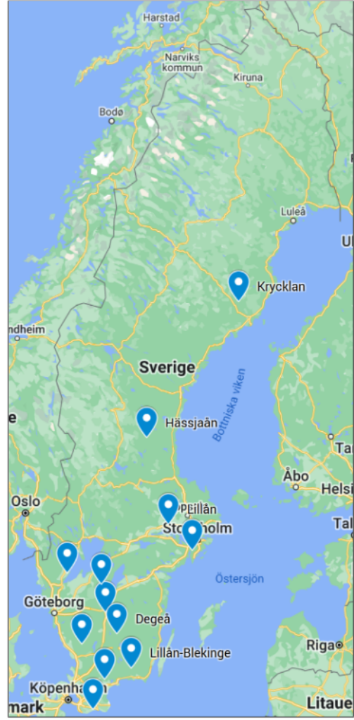
Fig. 1. The data used in this paper comes from 12 locations in Sweden: Jönköping (Tabergsån), Knislinge (Almaån), Krycklan, Skivarp (Skivarpsån), Skövde (Ösan), Torup (Kilan), Tumba (Saxbroån), Dalbergsån, Degeå, Hässjaån, Lillån, and Lillån-Blekinge. Note that Lillån and Lillån-Blekinge are far apart (Lillån is north-west of Stockholm).
