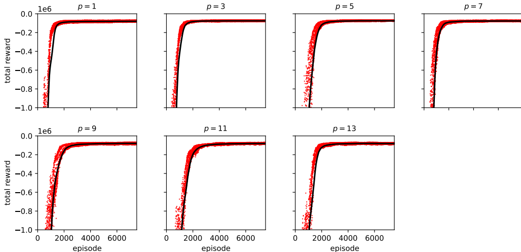
(b) Navier-Stokes
