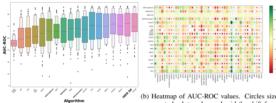
(a) Box plot presenting actual AUC-ROC values. RSR.
