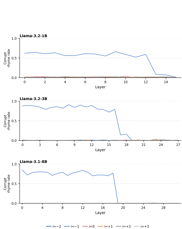
(d) Llama-3 1B–70B.
