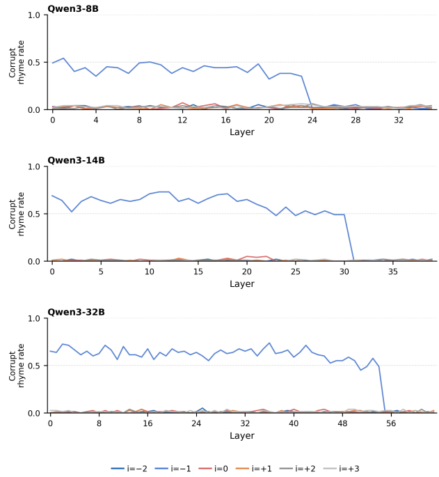
(b) Qwen3 8B–32B.
